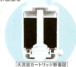
大流量カートリッジ断面図
